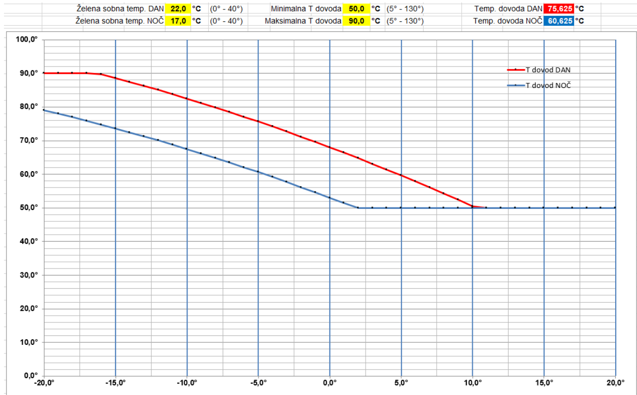
Priloga 1. Diagram poteka temperatur ogrevne vode v dovodnem in povratnem vodu na odjemnem mestu v odvisnosti od zunanjih temperatur
