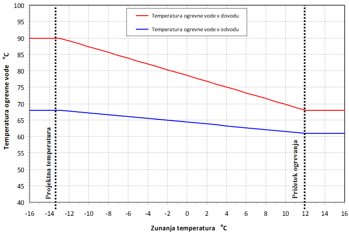
Priloga: Temperaturni diagram za zunanjo projektno temperaturo -13°C
