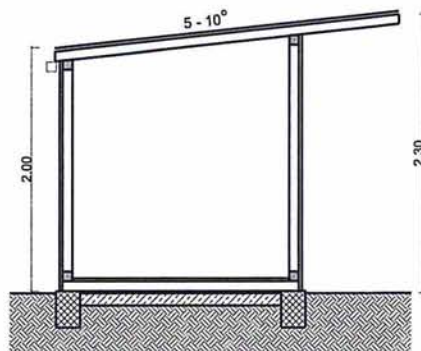
Prerez
