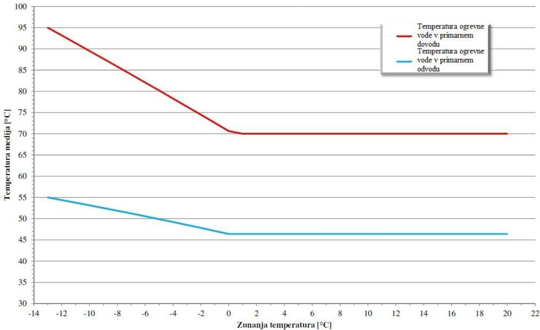
Priloga: Temperaturni diagram za zunanjo normno temperaturo -13^{\circ}\text{C}
