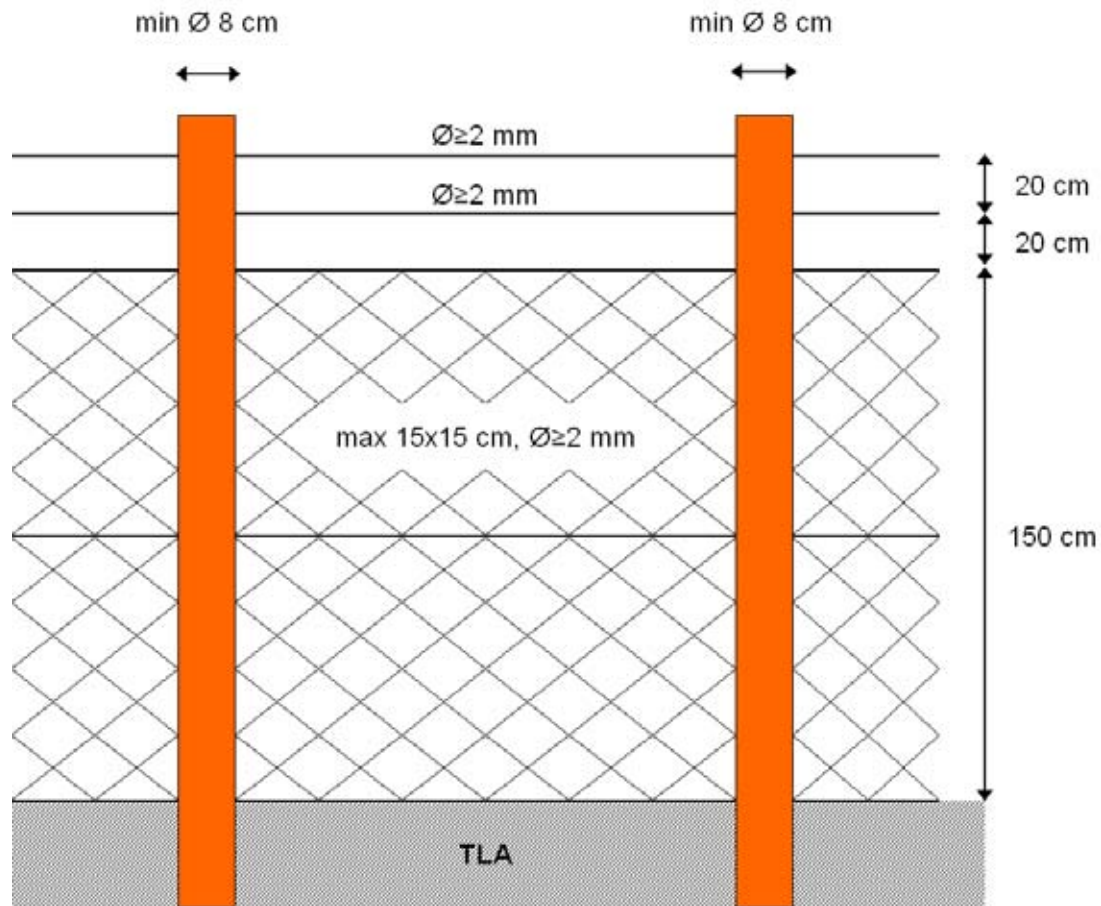
PRILOGA 1: Mreža ograje za zaščito pred navadnim jelenom, damjakom, gamsom in alpskim kozorogom
