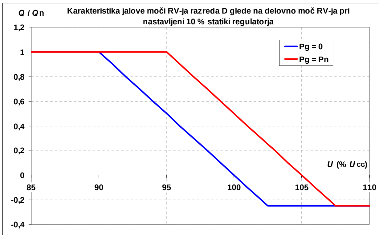
Slika 7.4: Karakteristika jalove moči razpršenih virov razreda D (do 10 MW vključeni v SN omrežje) pri nastavljeni 10 % statiki regulatorja jalove moči ( u_{STAT} = 0,1 ).
