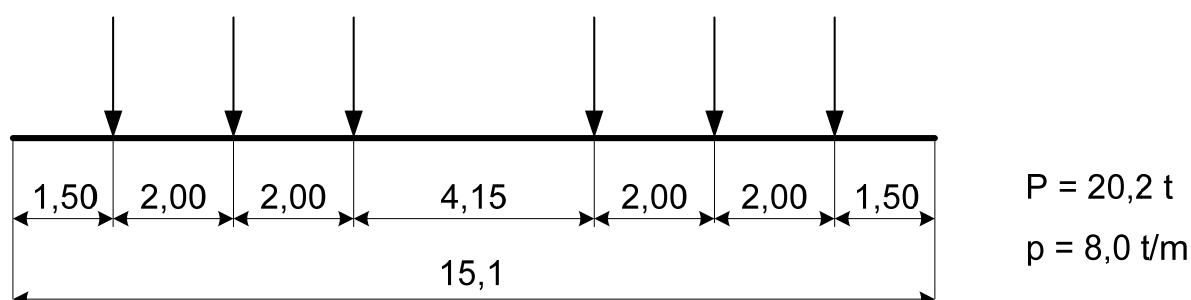
Vlečno vozilo CC
