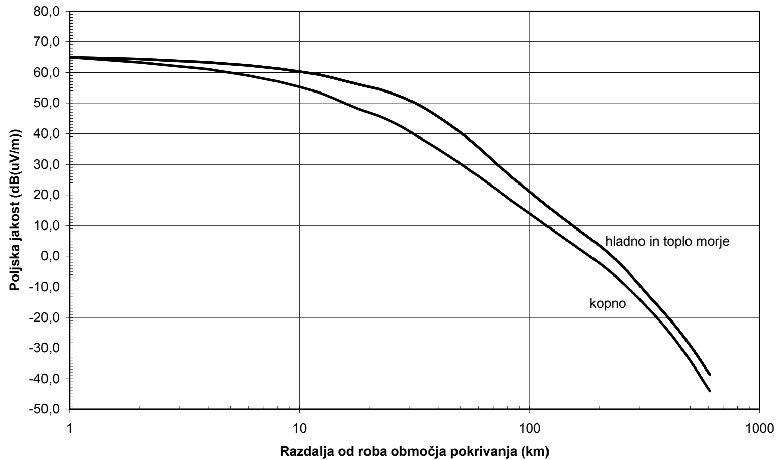
Slika 6a: Potencial motenja referenčnega omrežja ena za 50 % časa
