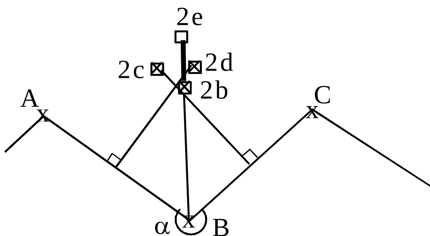
Slika 9: Postavitev dodatnih izračunskih preskusnih točk, če je \alpha \geq 180^\circ (glej spodnjo opombo)
