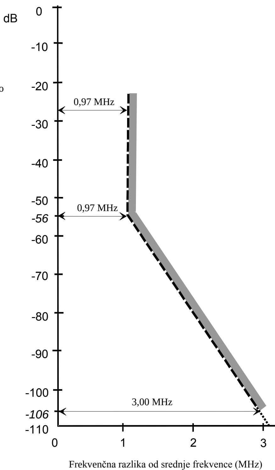
Slika 1: Spektralna maska za zunajpasovna oddajanja T-DAB
