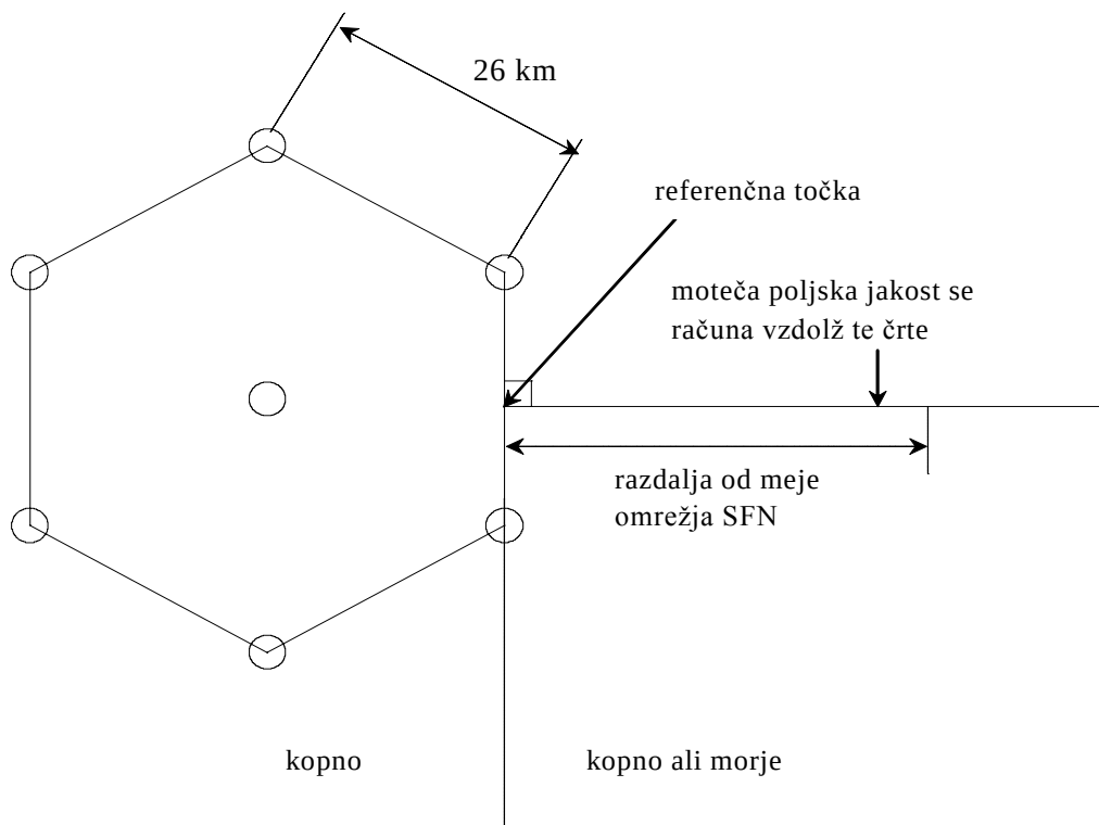
Slika 4: Diagram razporeda referenčnega omrežja dve
