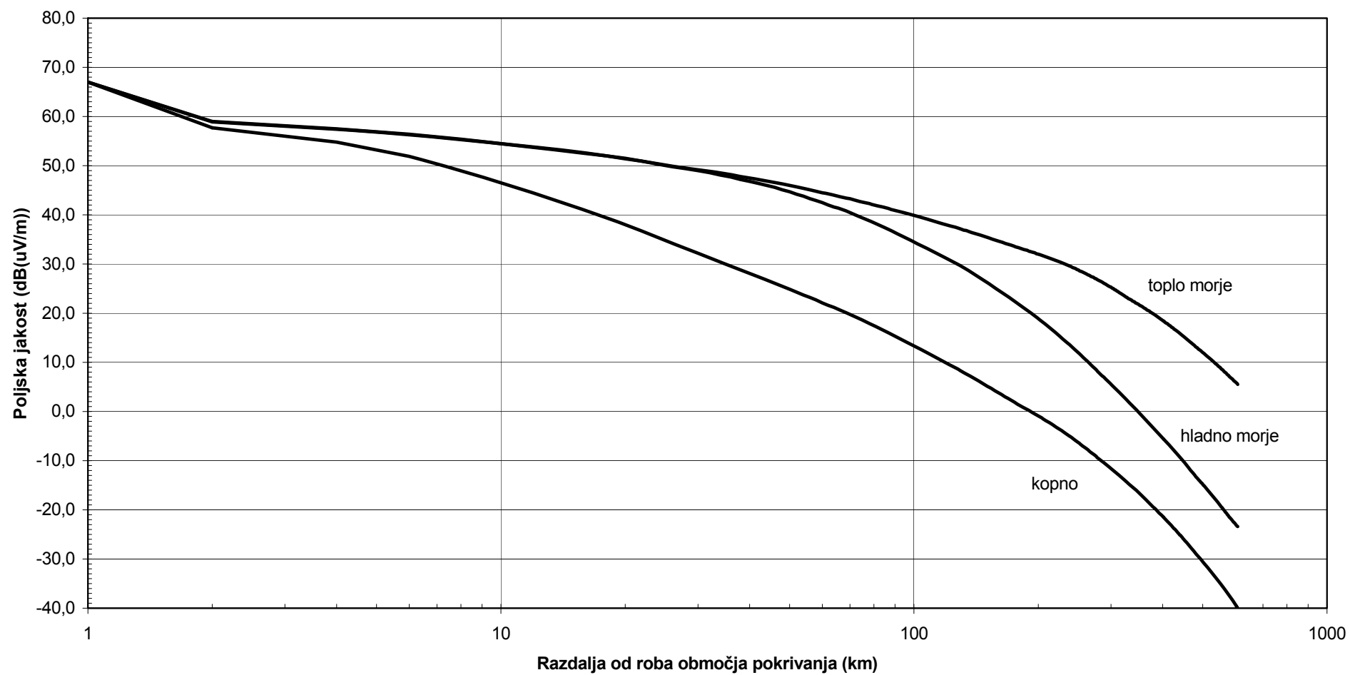
Slika 8b: Potencial motenja referenčnega omrežja tri za 1 % časa
