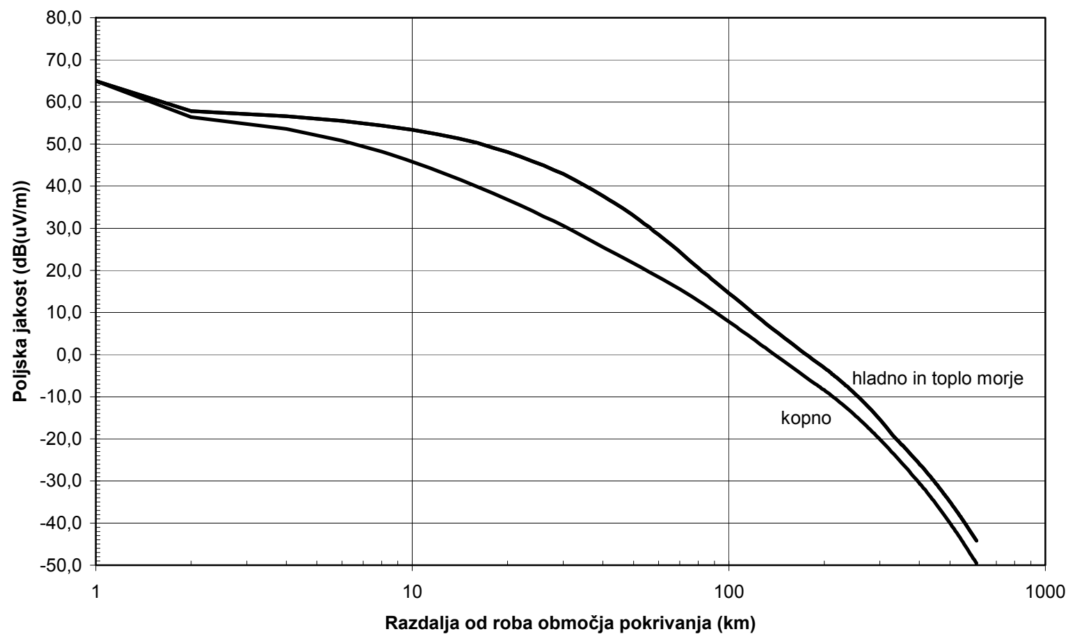
Slika 8a: potencial motenja referenčnega omrežja tri za 50 % časa
