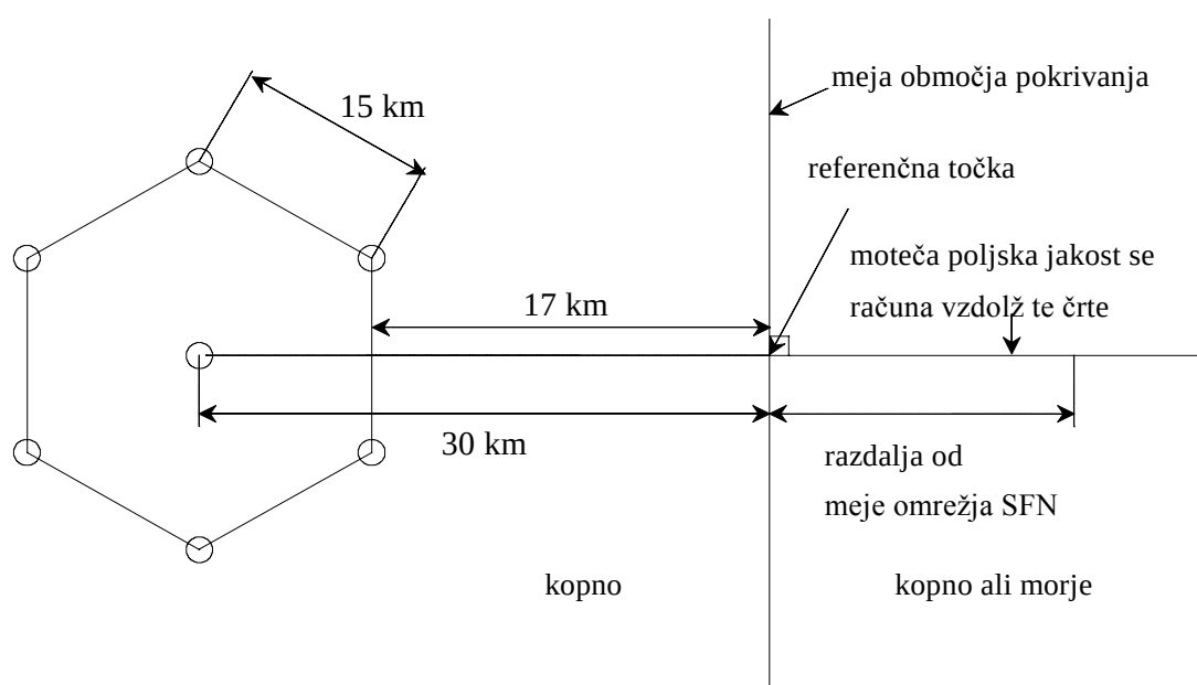
Slika 3: Diagram razporeda referenčnega omrežja ena
