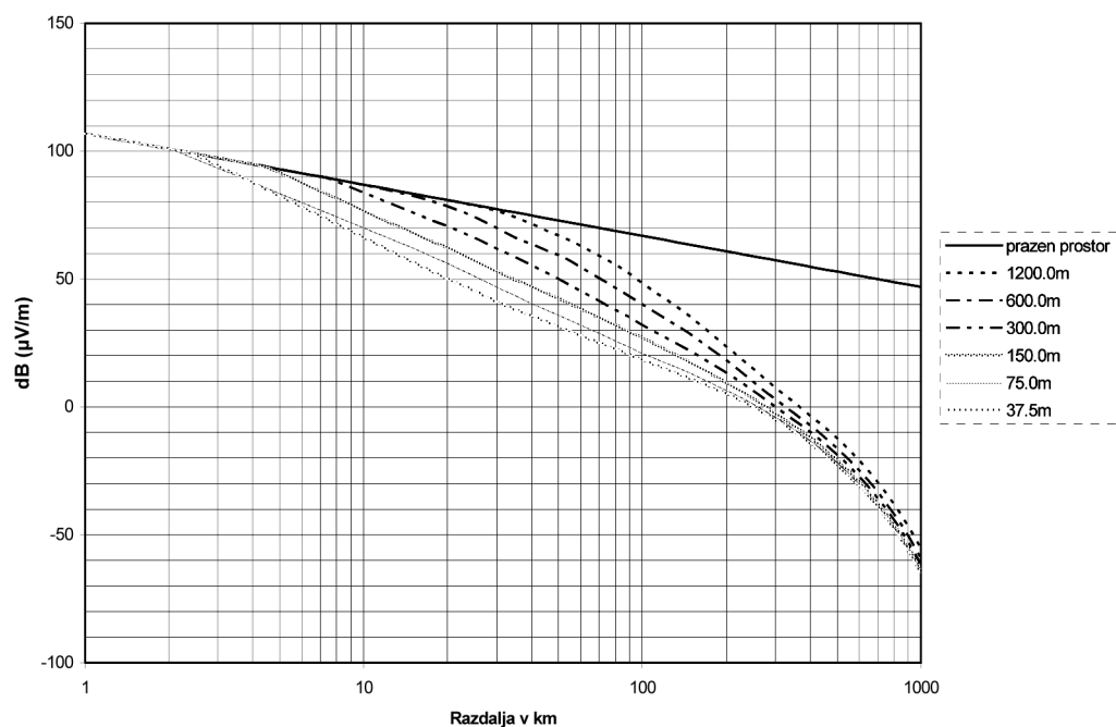
Slika 1b: Poljska jakost za 1 kW e.r.p. proti razdalji kot funkcija efektivne višine oddajne antene; KOPNO; 1 % časa
