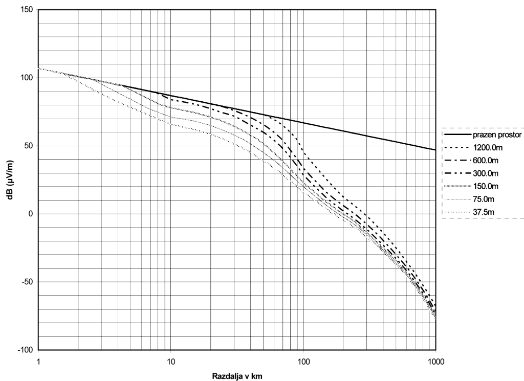
Slika 3a: Poljska jakost za 1 kW e.r.p. proti razdalji kot funkcija efektivne višine oddajne antene; TOPLO MORJE; 50 % časa
