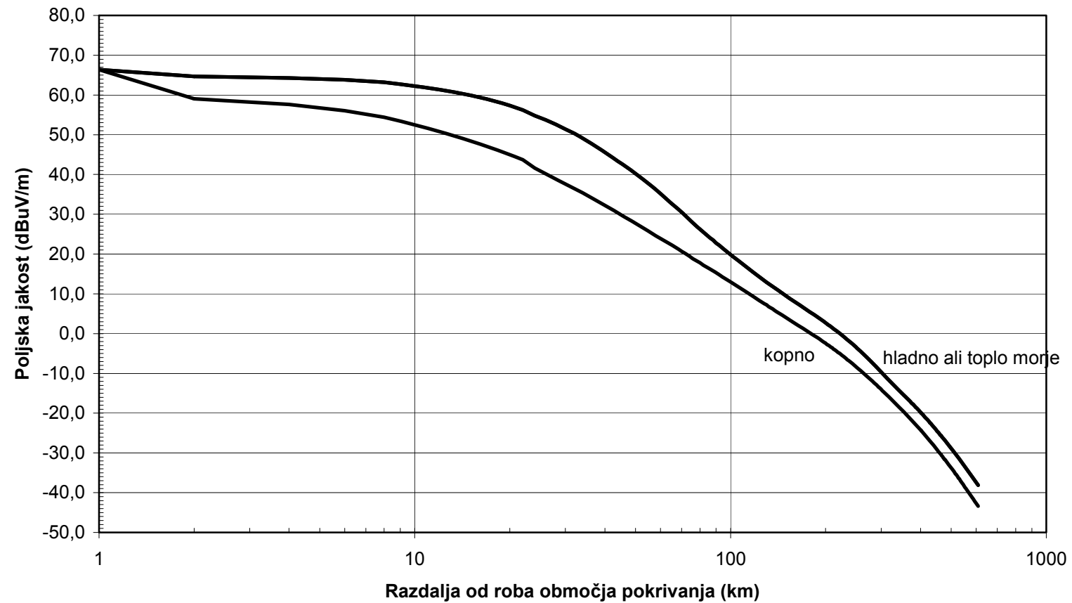
Slika 7a: Potencial motenja referenčnega omrežja dve za 50 % časa
