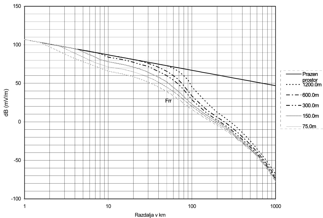
Slika 2a: Poljska jakost za 1 kW e.r.p. proti razdalji kot funkcija efektivne višine oddajne antene; HLADNO MORJE; 50 % časa
