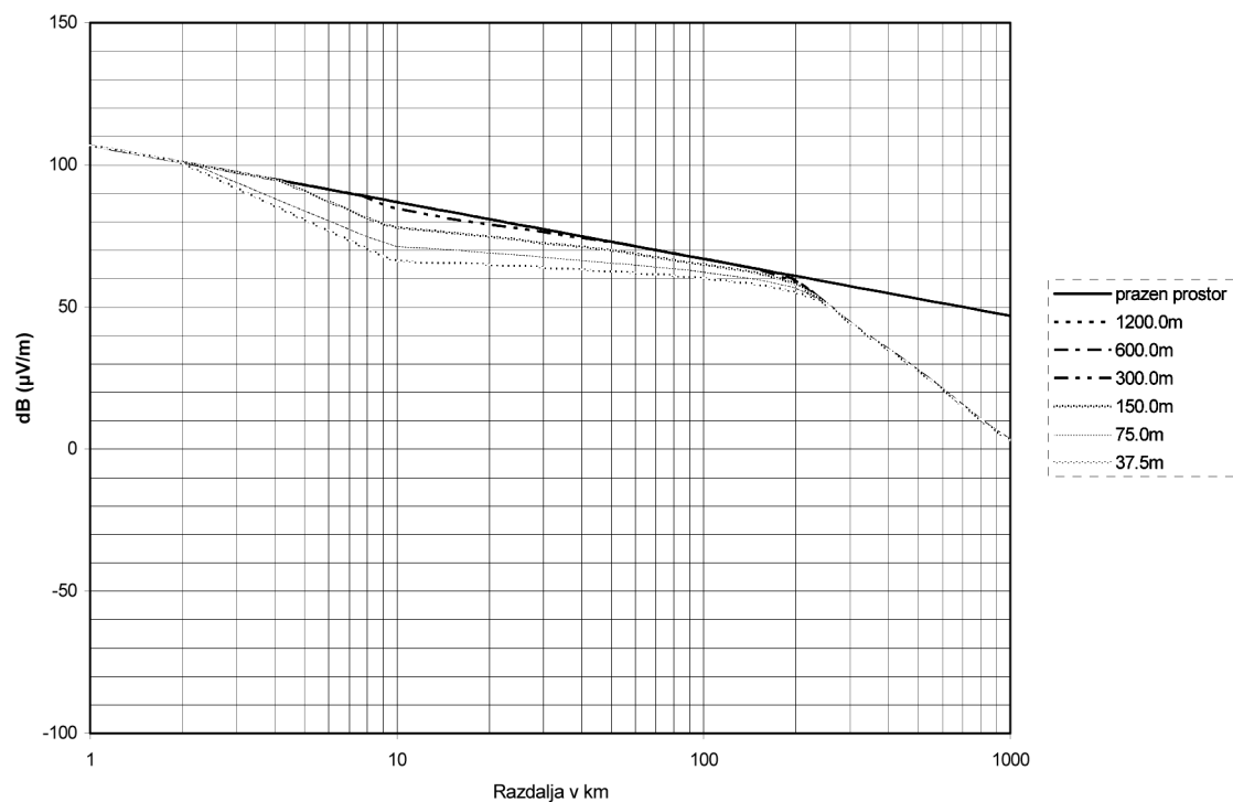
Slika 2b: Poljska jakost za 1 kW e.r.p. proti razdalji kot funkcija efektivne višine oddajne antene; HLADNO MORJE; 1 % časa
