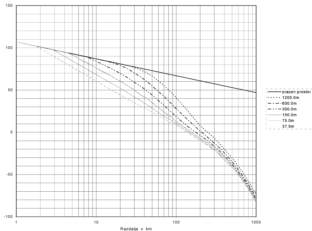
Slika 1a: Poljska jakost za 1 kW e.r.p. proti razdalji kot funkcija efektivne višine oddajne antene; KOPNO; 50 % časa
