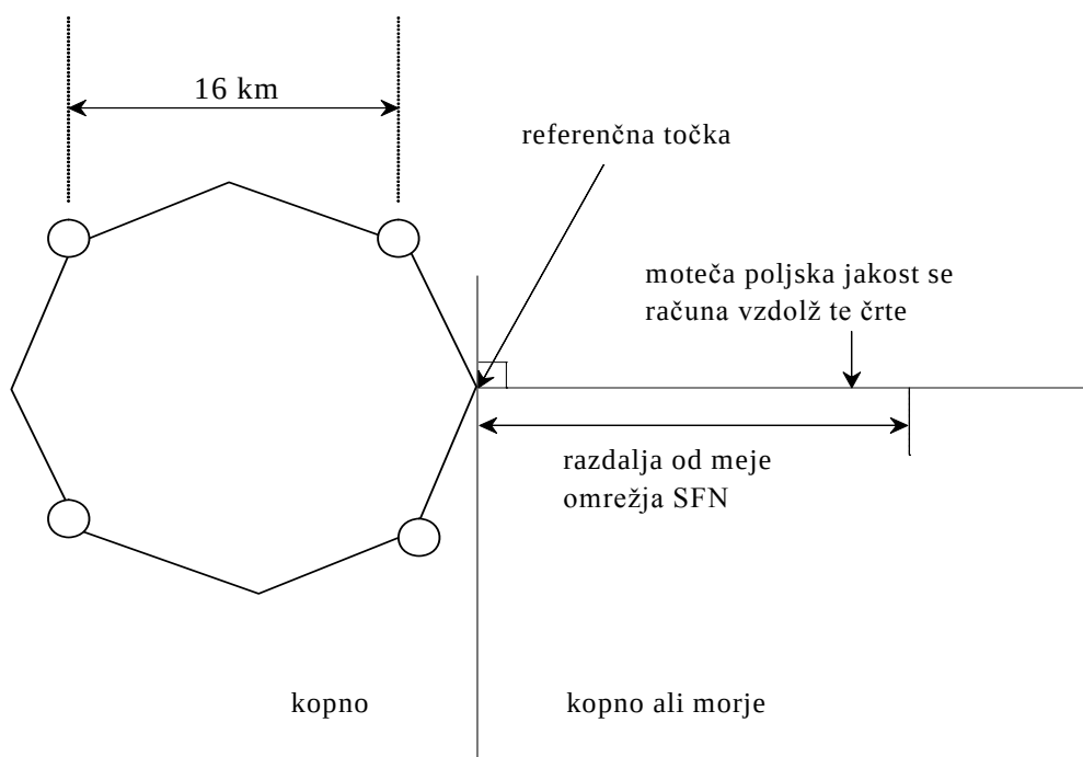
Slika 5: Diagram razporeda referenčnega omrežja tri
