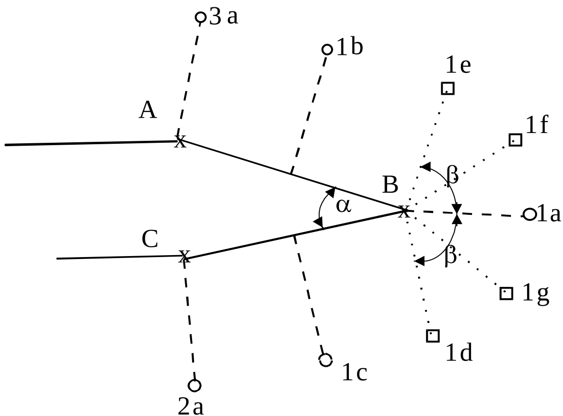
Slika 8: Postavitev dodatnih izračunskih preskusnih točk, če je \alpha < 180^\circ (glej spodnjo opombo)
