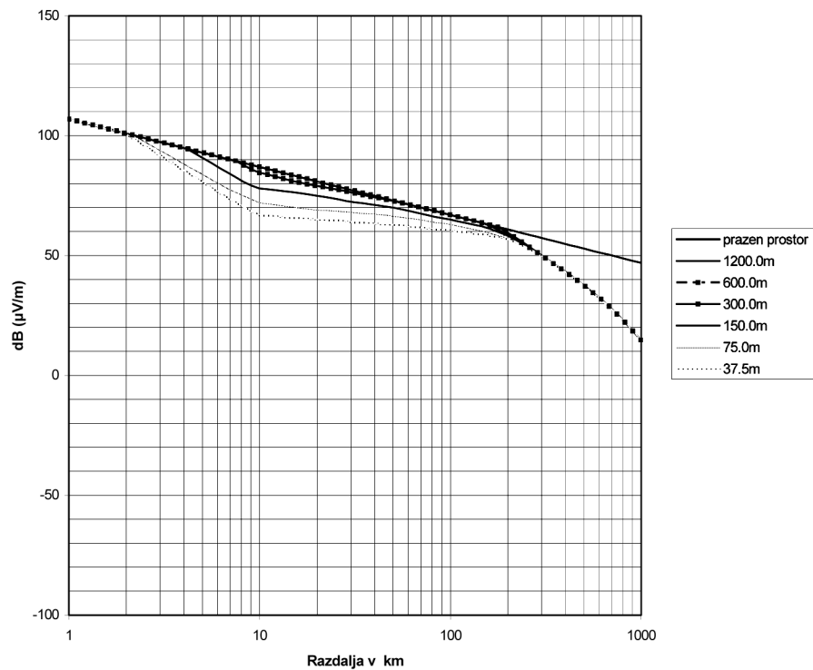
Slika 3b: Poljska jakost za 1 kW e.r.p. proti razdalji kot funkcija efektivne višine oddajne antene; TOPLO MORJE; 1 % časa
