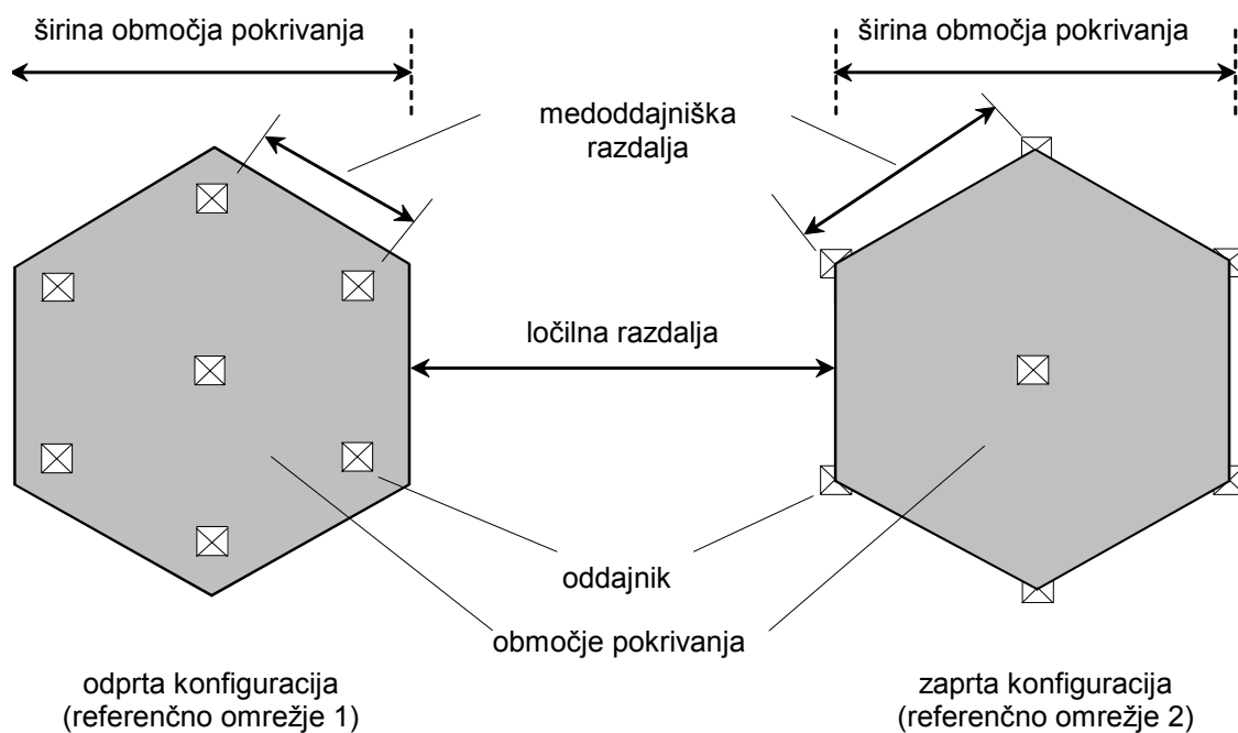
Slika 2: Primer struktur omrežij T-DAB in razdalj – primer sobloka
