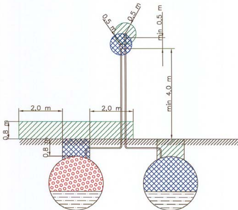
REZERVOAR Z BENCINOM
