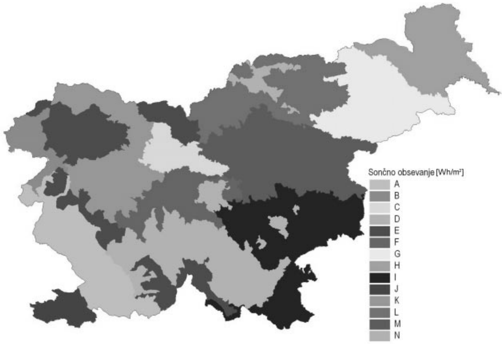
Karta 4 Karta območij globalnega sončnega obsevanja
