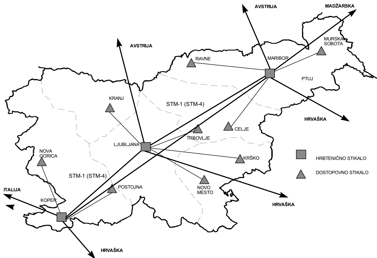
Slika 6.4.6 - Povezave dostopovnih stikal ATM ter hrbtničnih stikal in mednarodne povezave
