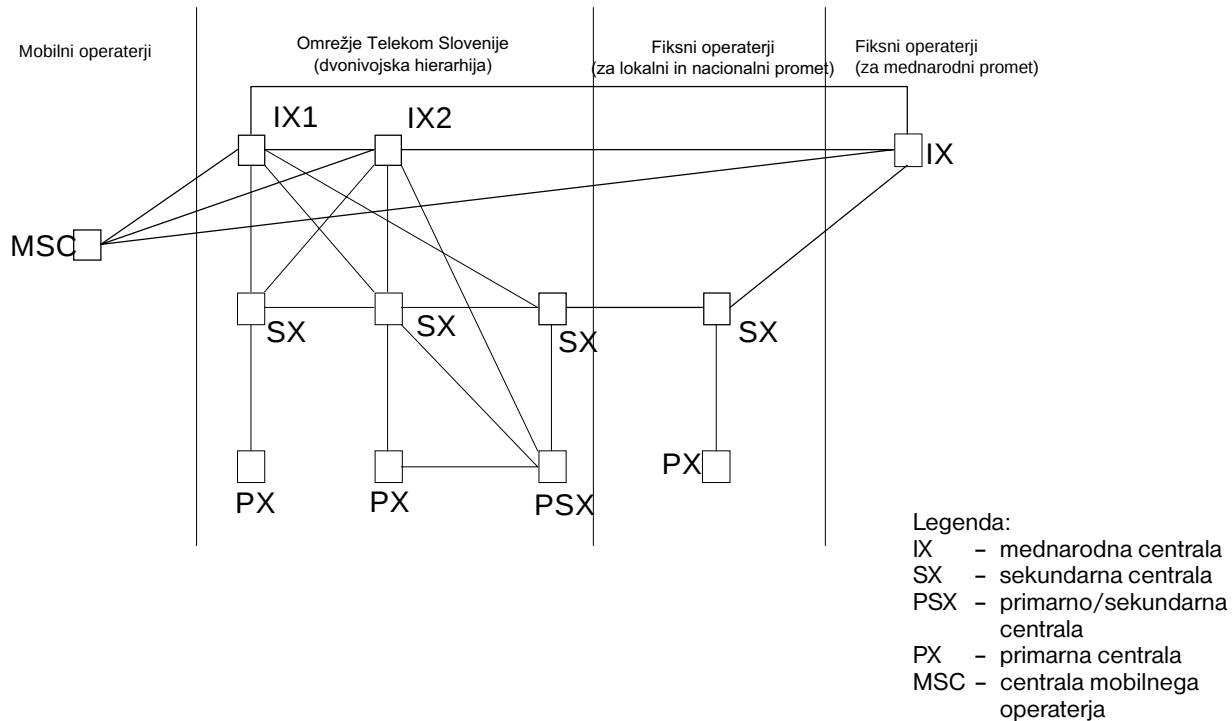
Slika 6.4.1 – Dvoravinska struktura central
