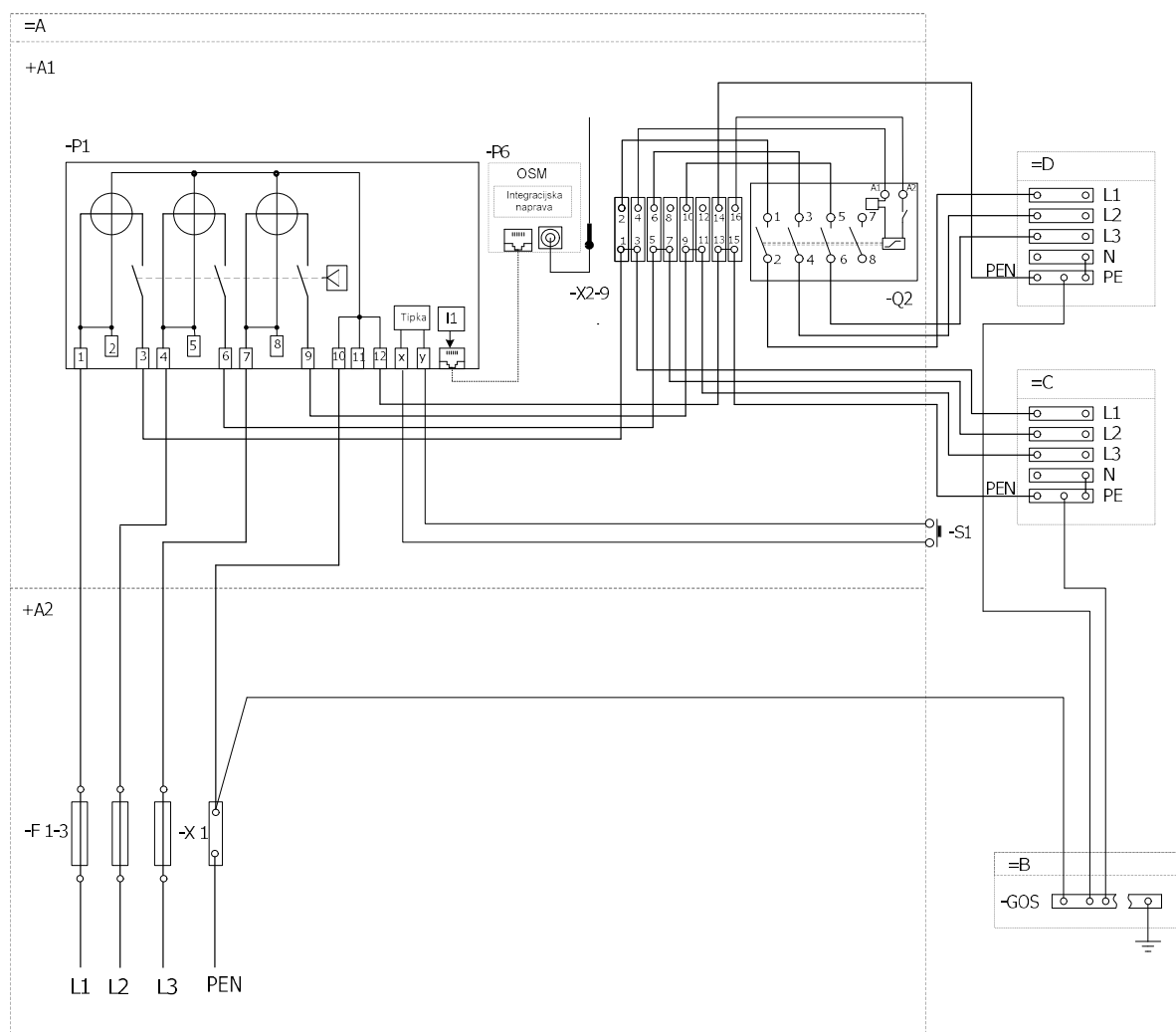
Slika 34a: Izvedba 2, sistem TN, z glavnimi varovalkami in stikalno napravo za omejevanje toka in priključeno napravo za samooskrbo v priključno-merilni omarici
