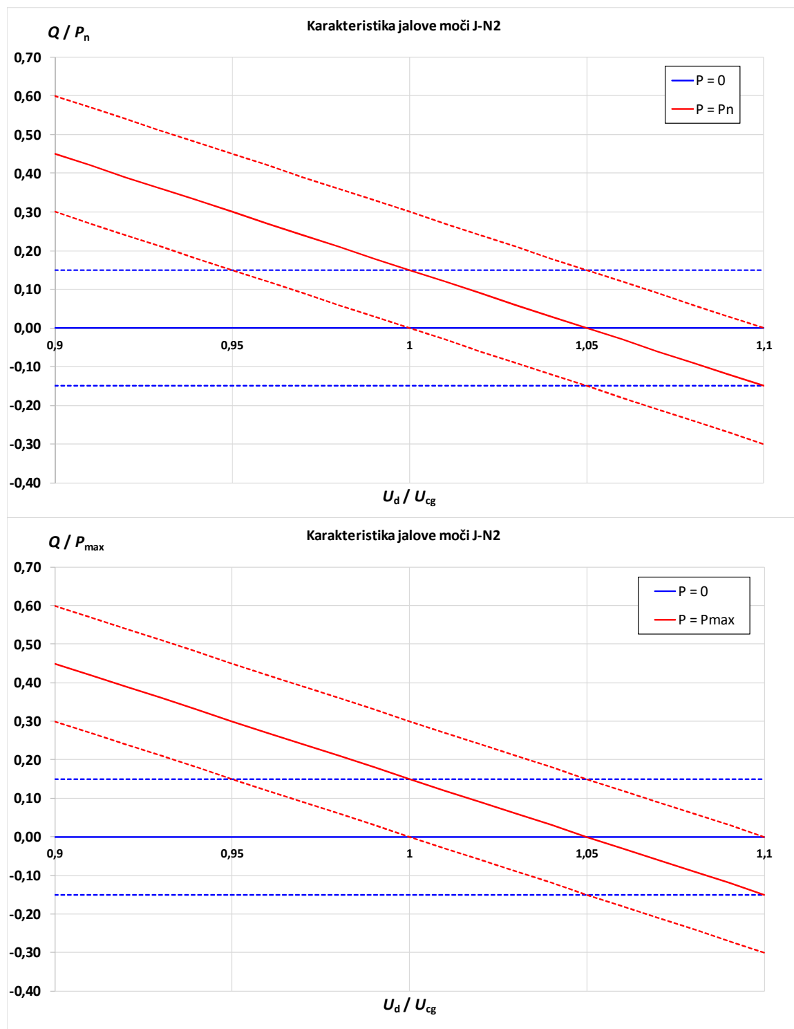
Slika XII.3: Grafični prikaz predpisane karakteristiko jalove moči J-N2.
