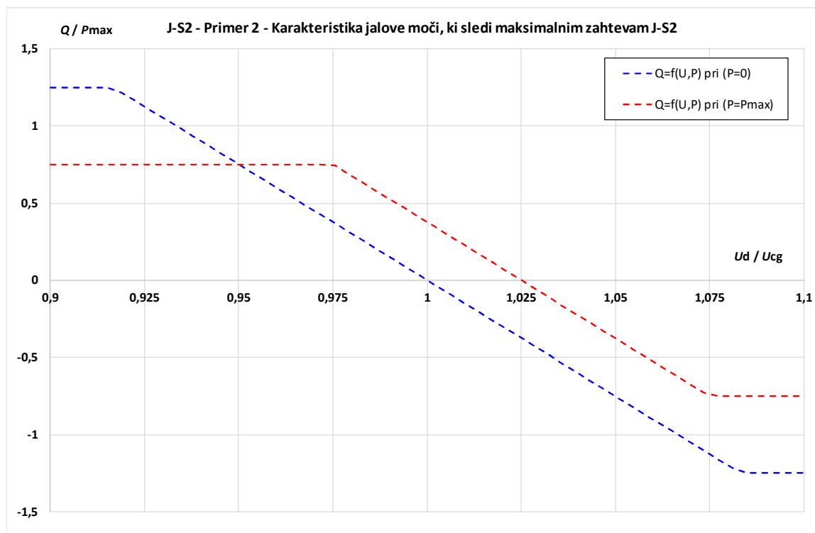
Slika XII.12: Grafični prikaz karakteristike jalove moči PN oziroma EM, ki (Primer 2) zagotavlja maksimalne zahteve glede jalove moči po karakteristiki J-S2.
