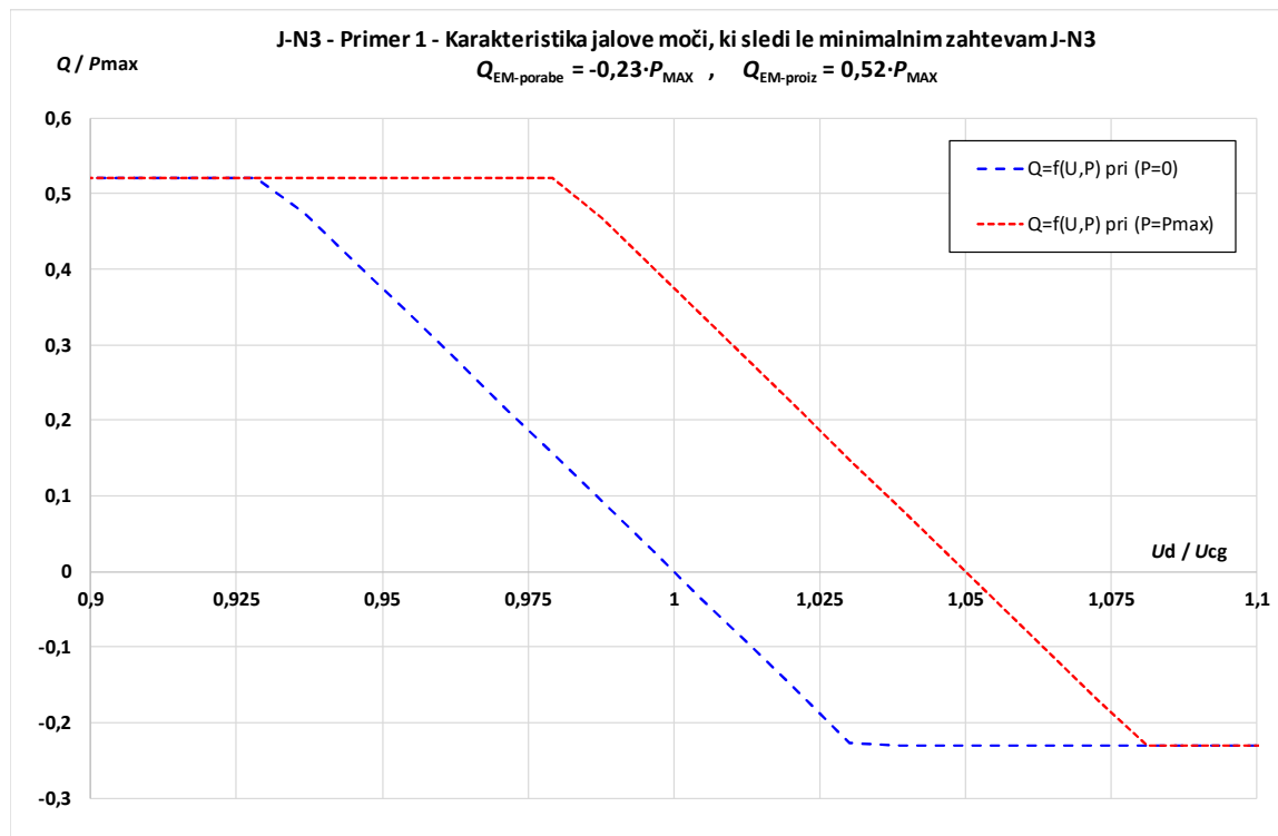
Slika XII.5: Grafični prikaz karakteristike jalove moči PN oziroma EM, ki (Primer 1) zagotavlja minimalne zahteve glede jalove moči po karakteristiki J-N3.
