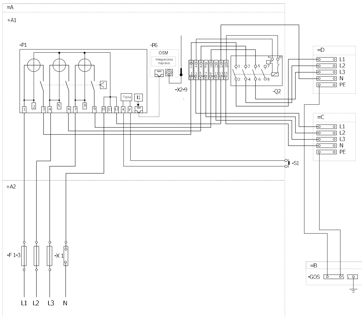
Slika 36a: Izvedba 2, sistem TT, z glavnimi varovalkami in stikalno napravo za omejevanje toka in priključeno napravo za samooskrbo v priključno-merilni omarici
