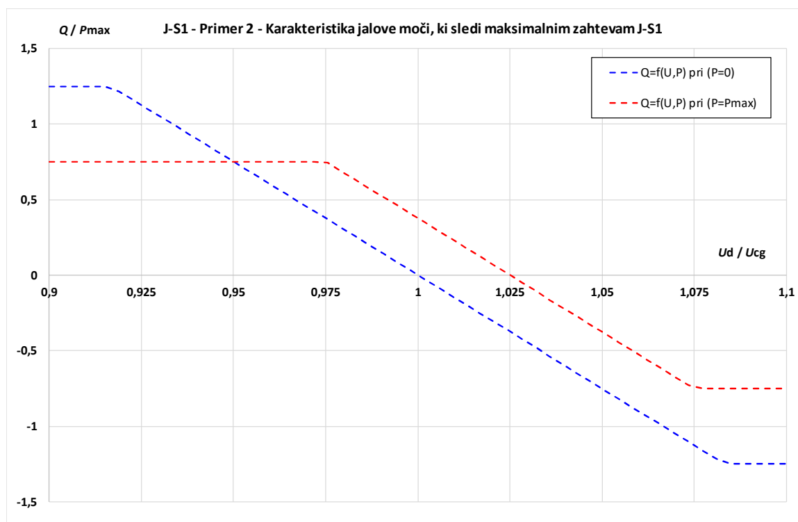
Slika XII.9: Grafični prikaz karakteristike jalove moči PN oziroma EM, ki (Primer 2) zagotavlja maksimalne zahteve glede jalove moči po karakteristiki J-S1.
