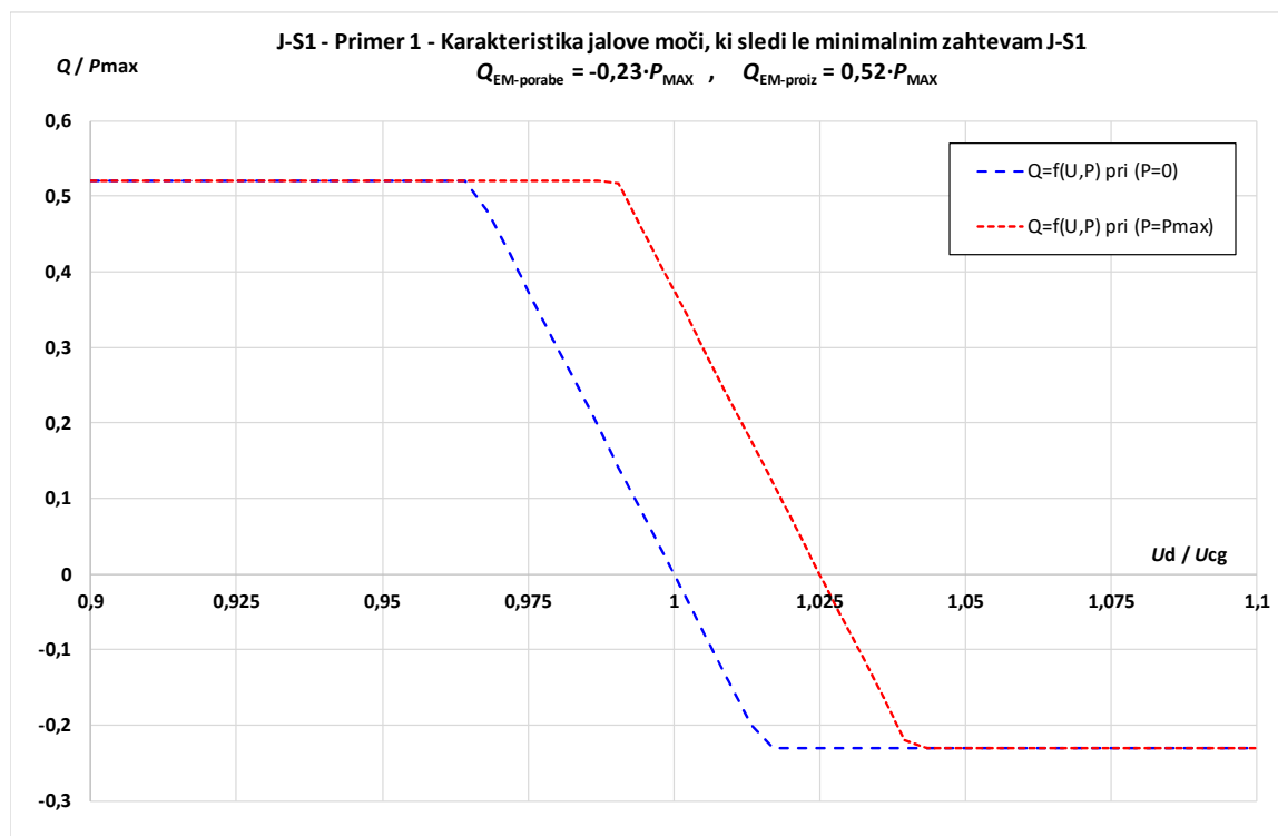
Slika XII.8: Grafični prikaz karakteristike jalove moči PN oziroma EM, ki (Primer 1) zagotavlja minimalne zahteve glede jalove moči po karakteristiki J-S1.
