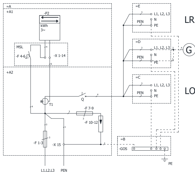
Slika 22: Polindirektni način, izvedba 1, shema priključitve PS 1
