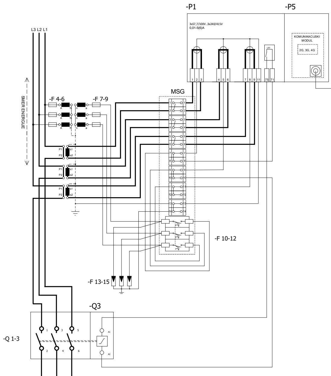
Slika 42: Izvedba 5 Omejevanje moči
