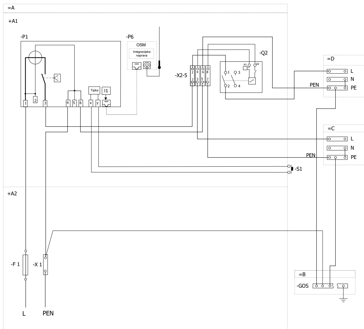
Slika 30a: Izvedba 1, sistem TN, z glavno varovalko in stikalno napravo za omejevanje toka in priključeno napravo za samooskrbo v priključno-merilni omarici
