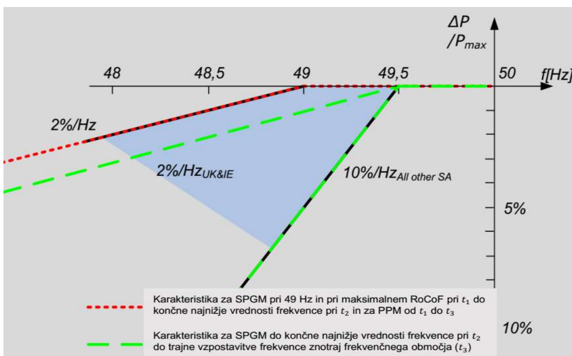
Slika IX.1: Največje dopustno zmanjšanje delovne moči iz največje izhodne delovne moči glede na padajočo frekvenco. Oznaka SPGM na sliki pomeni SPGM.
