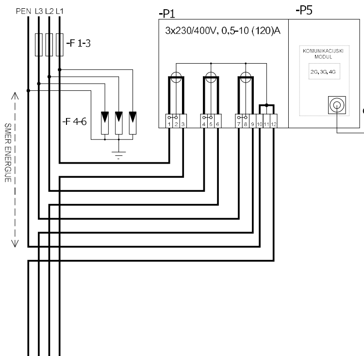
Slika 37: Izvedba 3, sistem TN
