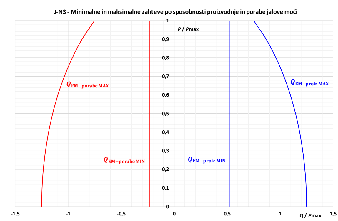
Slika XII.4: Grafični prikaz minimalnih in maksimalnih zahtev glede proizvodnje in porabe jalove moči J-N3.
