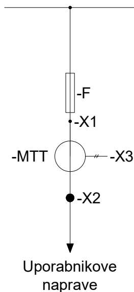
Slika 3: Način priključitve merilnega mesta
