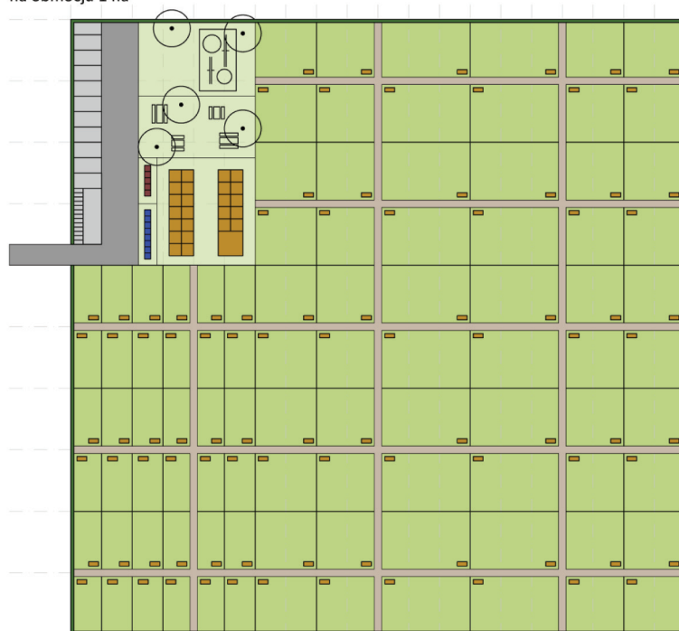
7. Primer tipske ureditve območja vrtnikov s skupnim objektom za shranjevanje orodja na območju 1 ha
