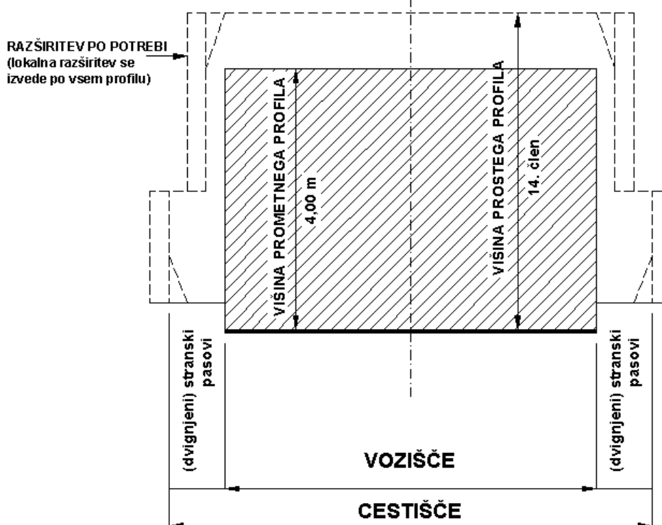
Slika IV-1: Sestavni deli cestišča v predoru, elementi prečnega profila
