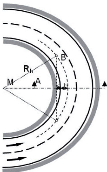
Slika III-1: Shema za preveritev preglednosti v enosmerni predorski cevi (povzeto po: RAS-L, 1995)
