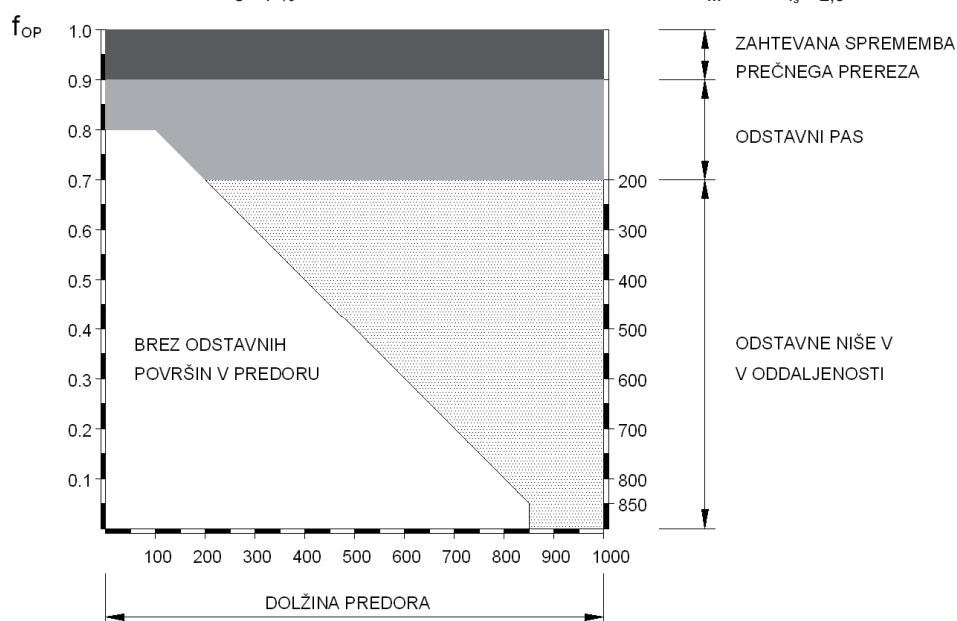
Slika IV-2: Razpored in medsebojna oddaljenost odstavnih površin za predore brez naprav za krmiljeno vodenje prometa (povzeto po RVS 9.232)
