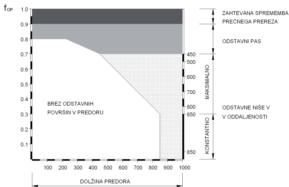
Slika IV-3: Razpored in medsebojna oddaljenost odstavnih površin za predore z napravami za krmiljeno vodenje prometa (povzeto po RVS 9.232)
