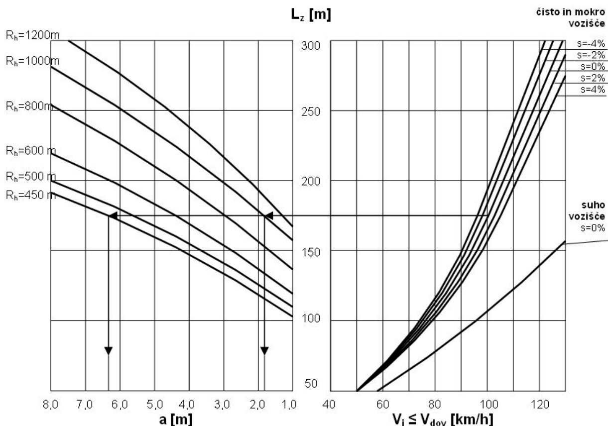
Slika III-2: Soodvisnost polmera R_h , razdalje a , hitrosti V_i in nagiba nivelete s (povzeto po: RAS-L, 1995)
