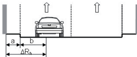
Slika III-1: Shema za preveritev preglednosti v enosmerni predorski cevi (povzeto po: RAS-L, 1995)
