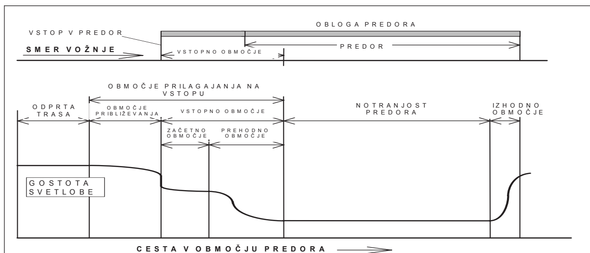
Slika XIV-1: Shematični prikaz poteka gostote svetlobe pri vožnji skozi predor – podnevi
