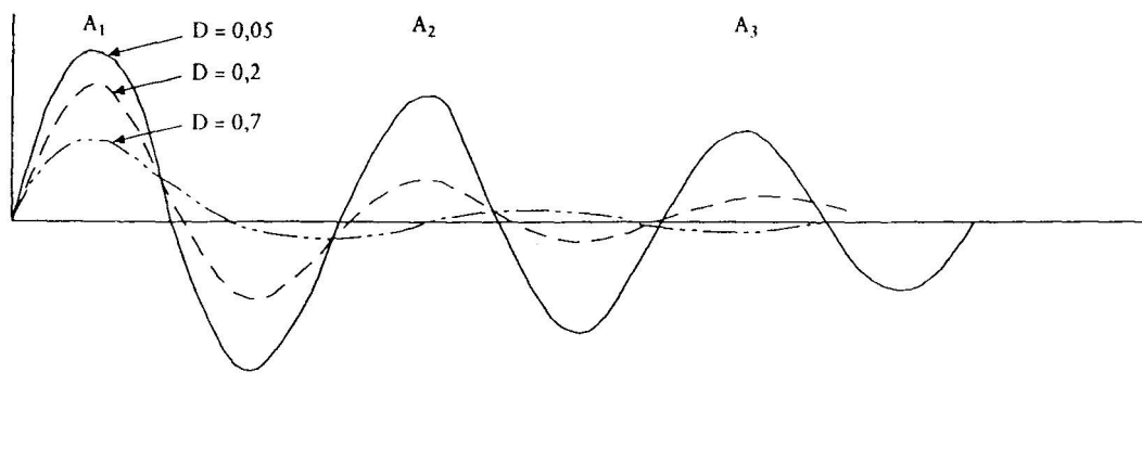
Slika 2 Prehodno dušeno nihanje čas
