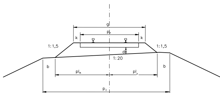
Prečni presek tirne grede v premi in enostranskem nagibu planuma
