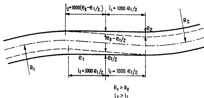
Razširjenje tira v S-krivinah z različnima krožnima lokoma
