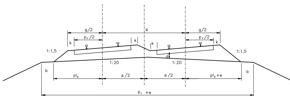
Prečni presek tirne grede dvotirne proge v loku
