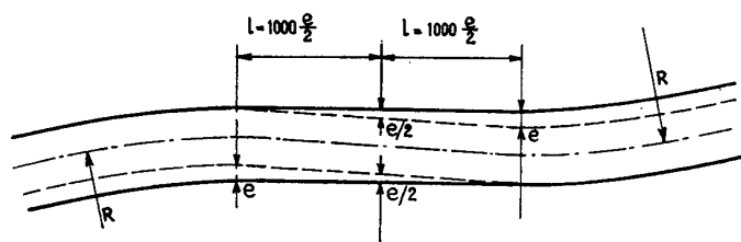
Razširjenje tira v S-krivinah z enakima krožnima lokoma
