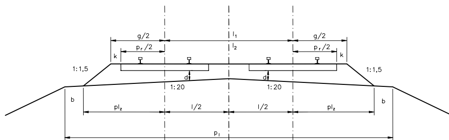
Prečni presek tirne grede dvotirne proge v premi
