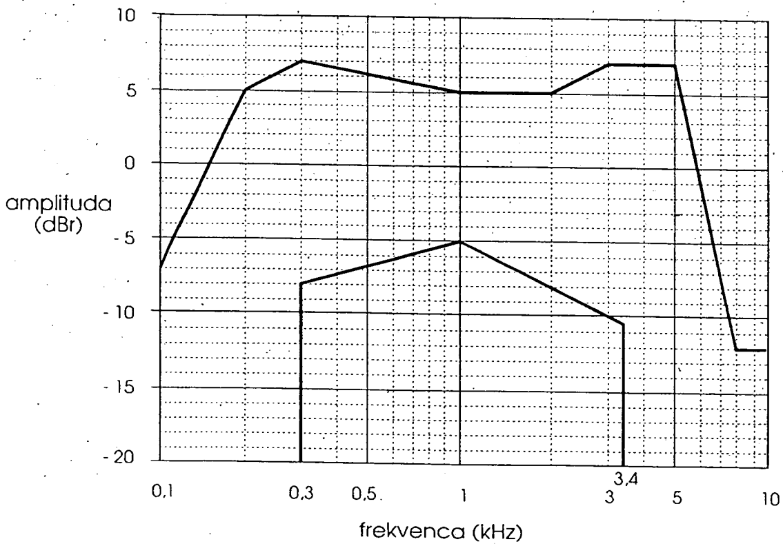
Risba 2: amplitudna karakteristika sprejema
