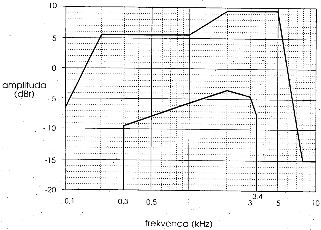
Risba 1: amplitudna karakteristika oddaje
